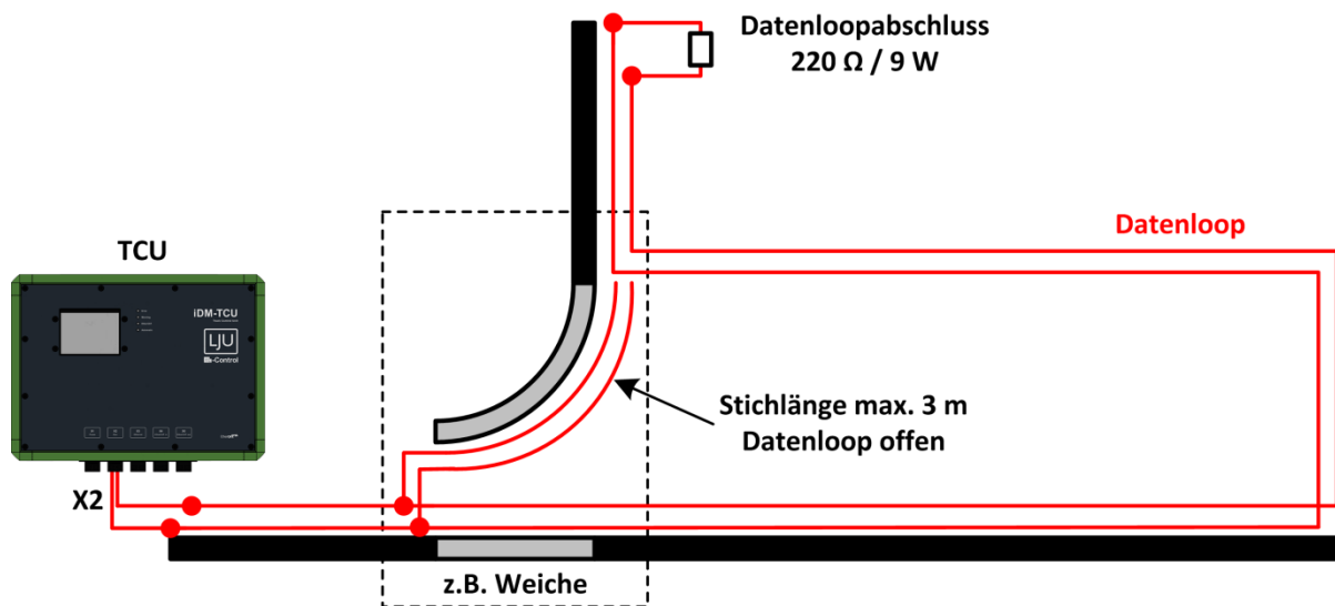
Abbildung 2: Datenloopverlegung
